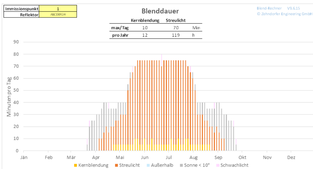
Abbildung 18 Blenddauer (mit Maßnahmen)
