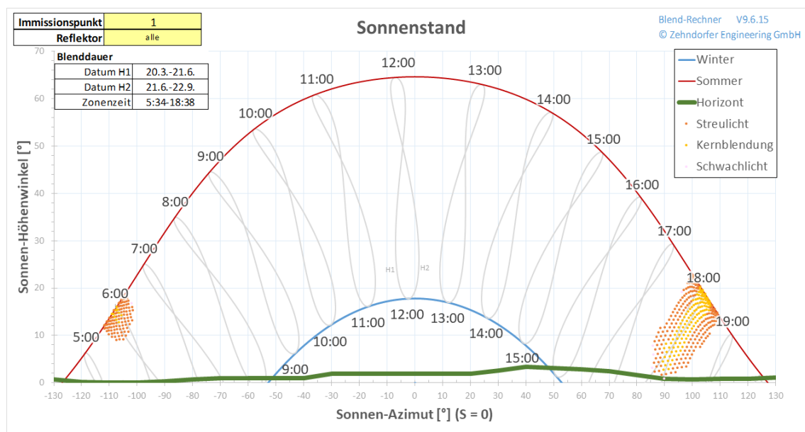
Abbildung 9 Sonnenwinkel bei Blendung
